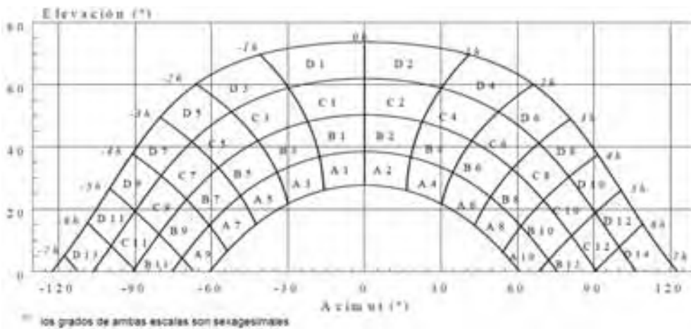
Figura 5. Diagrama de trayectorias del sol.
