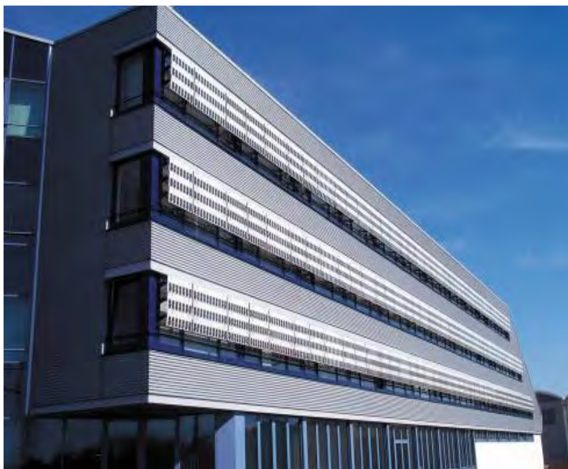
Foto 24. Instalación FV integrada en los parasoles en Eschweiler (Alemania).
